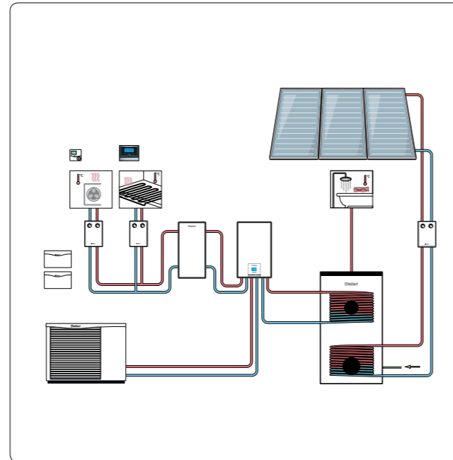
Dizalica topline aroTHERM u kombinaciji sa solarnim sustavom, hidrauličkom stanicom te međuspremnikom ogrjevnje /rashladne vode
